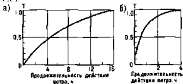
Рисунок 3 - Изменение коэффициента T в зависимости от продолжительности действия ветра в прибрежной мелководной (а) и глубоководной (б) зонах моря
