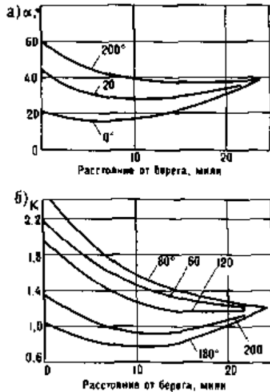
Рисунок 2 - Изменение угла \alpha отклонения направления поверхностных течений (а) и ветрового коэффициента К (б) в зависимости от направления ветра относительно берега и расстояния от него (приглубая зона)
