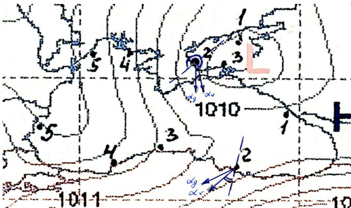
Рисунок 4 - Рабочая вырезка карты приземного атмосферного давления и температуры воздуха за 24 августа 2013 года с точками вариантов 16-20.
